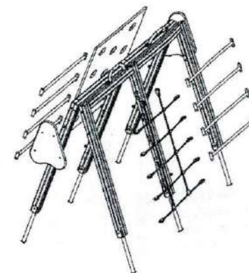
Elements assembling sandbox (Общая схема сборки элементов комплекса)
