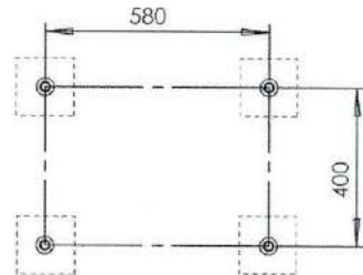
Scheme of placing of the foundation (Схема расположения фундаментов)
