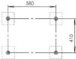
Scheme of placing of the foundation (Схема расположения фундаментов)
