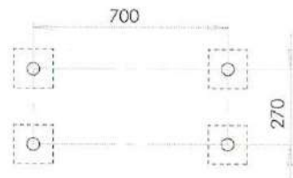
Scheme of placing of the foundation (Схема расположения фундаментов)
