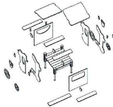
The elements fixation scheme (Схема крепления деталей)
