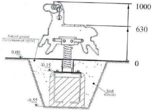
The equipment mounting plan (Схема монтажа оборудования)
